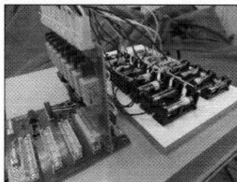
Foto 3: Ensaio de duração mínima/descarga Laboratório Labelo
