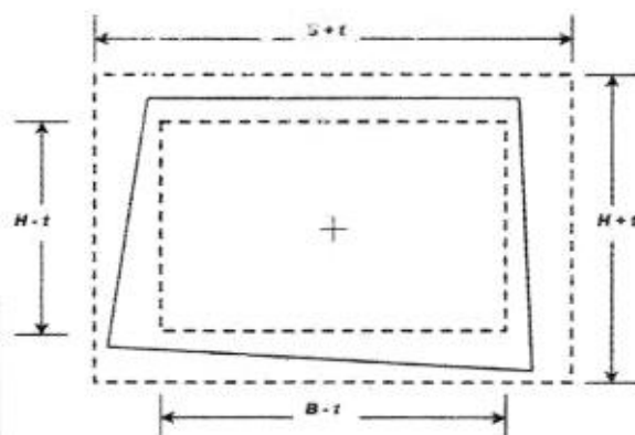
Figura 2 - Limites de tolerância para dimensões de chapas retangulares
